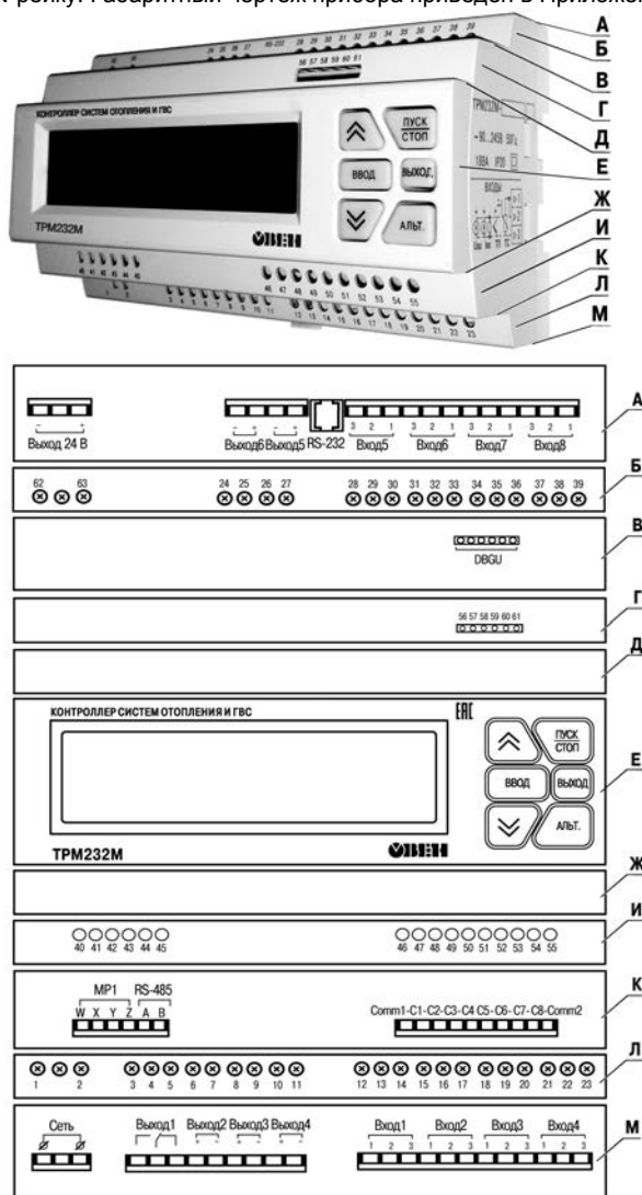
Рисунок 3.1 – Прибор TRM232M: клеммники, элементы индикации и управления
