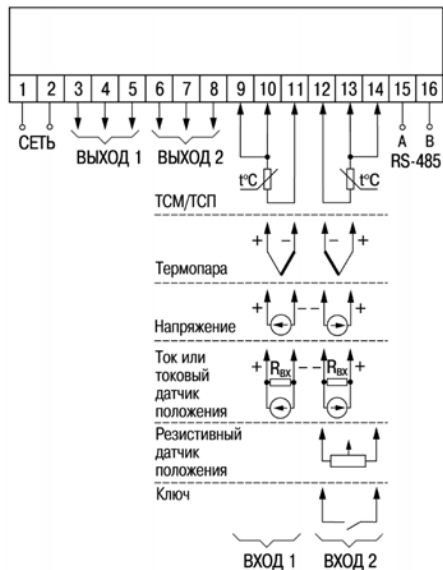
Рисунок Б.1 – Общая схема подключения TRM212-H, -Щ и -Щ2
