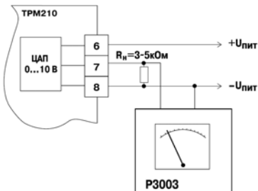
Рисунок Ж.7 – Подключение ВУ2 типа У
