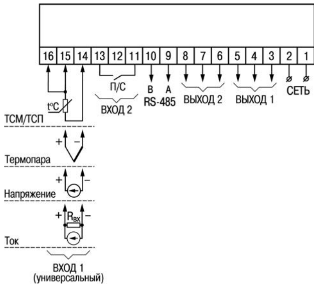
Рисунок Б.2 – Общая схема подключения TRM210-H2
