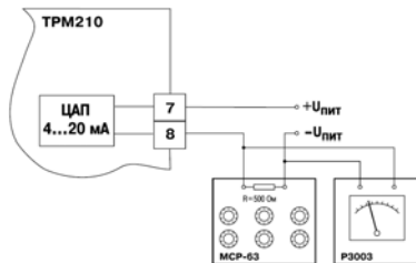
Рисунок Ж.5 – Подключение ВУ2 типа И
