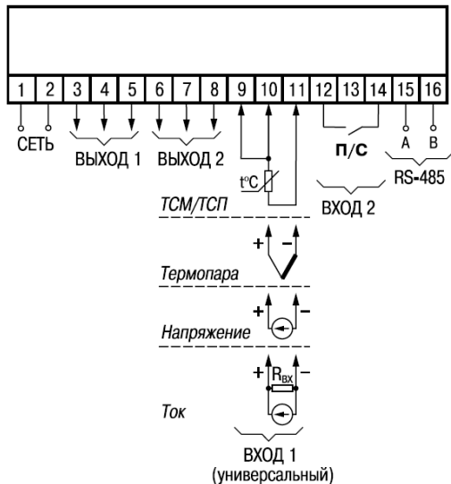
Рисунок Б.1 – Общая схема подключений TRM210-Н, Щ1 и Щ2
