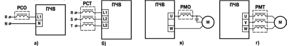
Рисунок 5.1 - Схемы подключения реакторов: а) серии PCO во входных цепях питания ПЧВ с однофазным входом; б) серии PCT во входных цепях питания ПЧВ с трехфазным входом; в) серии PMO в выходных цепях ПЧВ для питания однофазных электродвигателей; г) серии PMT в выходных цепях ПЧВ для питания трехфазных электродвигателей.
