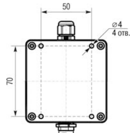
Рисунок А.2 – Монтажные отверстия
