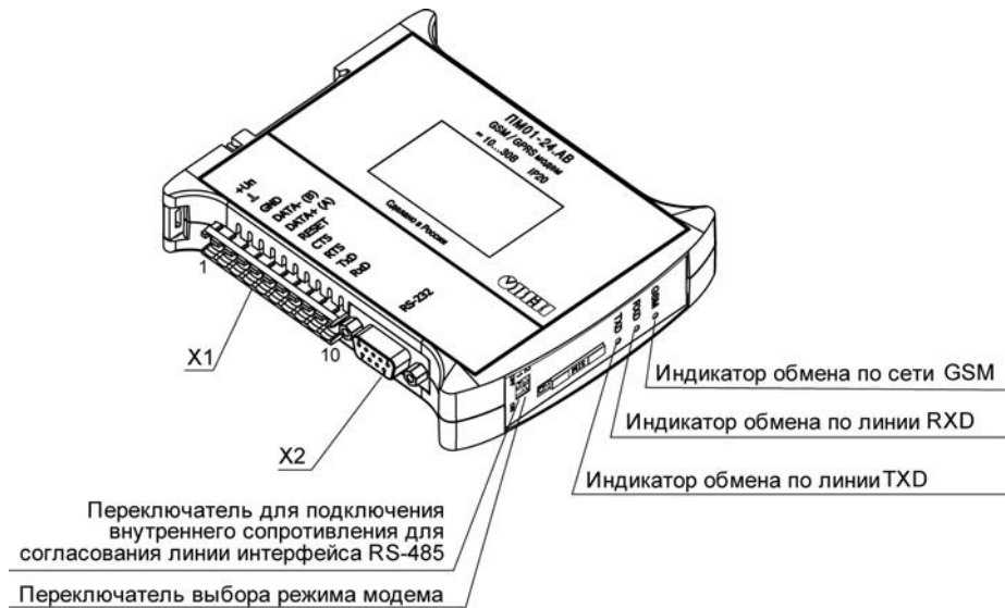
Рисунок 3.2 – Внешний вид модема
