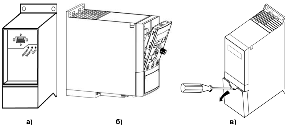
Рисунок 3.3 – Лицевая панель корпуса прибора: а) отсек ЛПО, б) установка ЛПО, в) клеммный отсек
