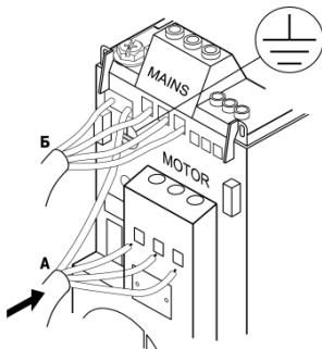
Рисунок 4.2 – Подключение:
