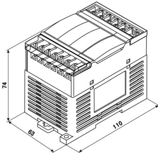
Рисунок А.1 - Габаритный чертеж МВ110
