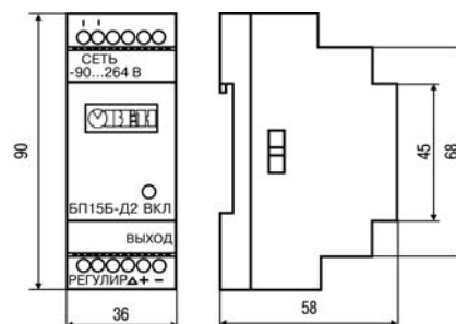
Рисунок 3.1 – Габаритные размеры блока питания БП15Б-Д2-х
