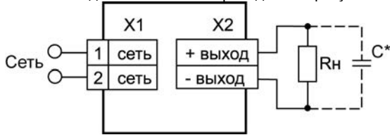
Рисунок 5.1 – Типовая схема подключения блока питания БП15Б-Д2-х
